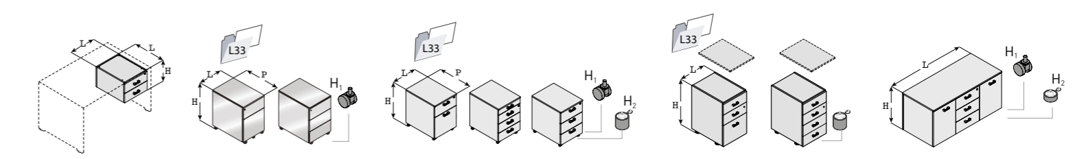
P 52,5 x H 31,5 L 42 P 53,5 x H 55,5 L 42 P 56 x H1/ H2 60 L 42 P 60 x H 72 L 42,5 P 55 x H+H1=58; H+H2= 60,5 L 120
